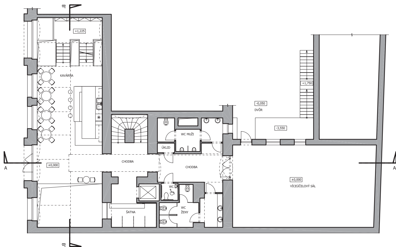
PŮDORYS 1. NP M 1:200
