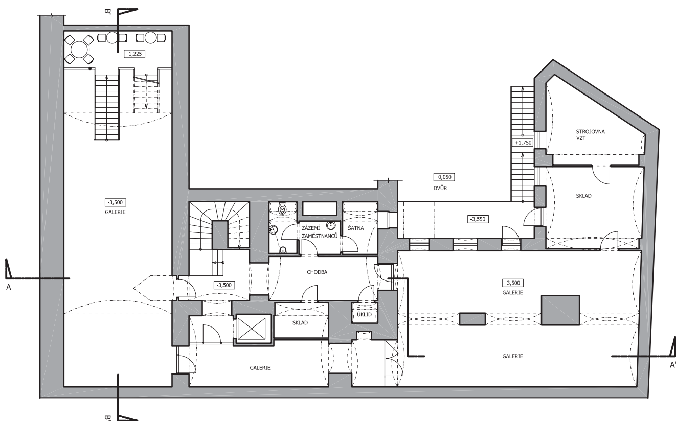
PŮDORYS 1. PP M 1:200
