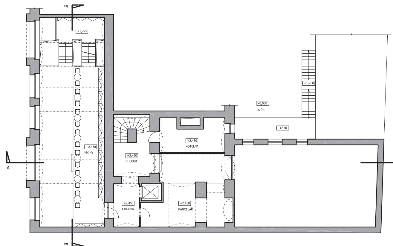
PŮDORYS MEZIPATRA M 1:200
